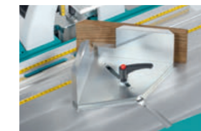
Butée centrale avec rehausse
