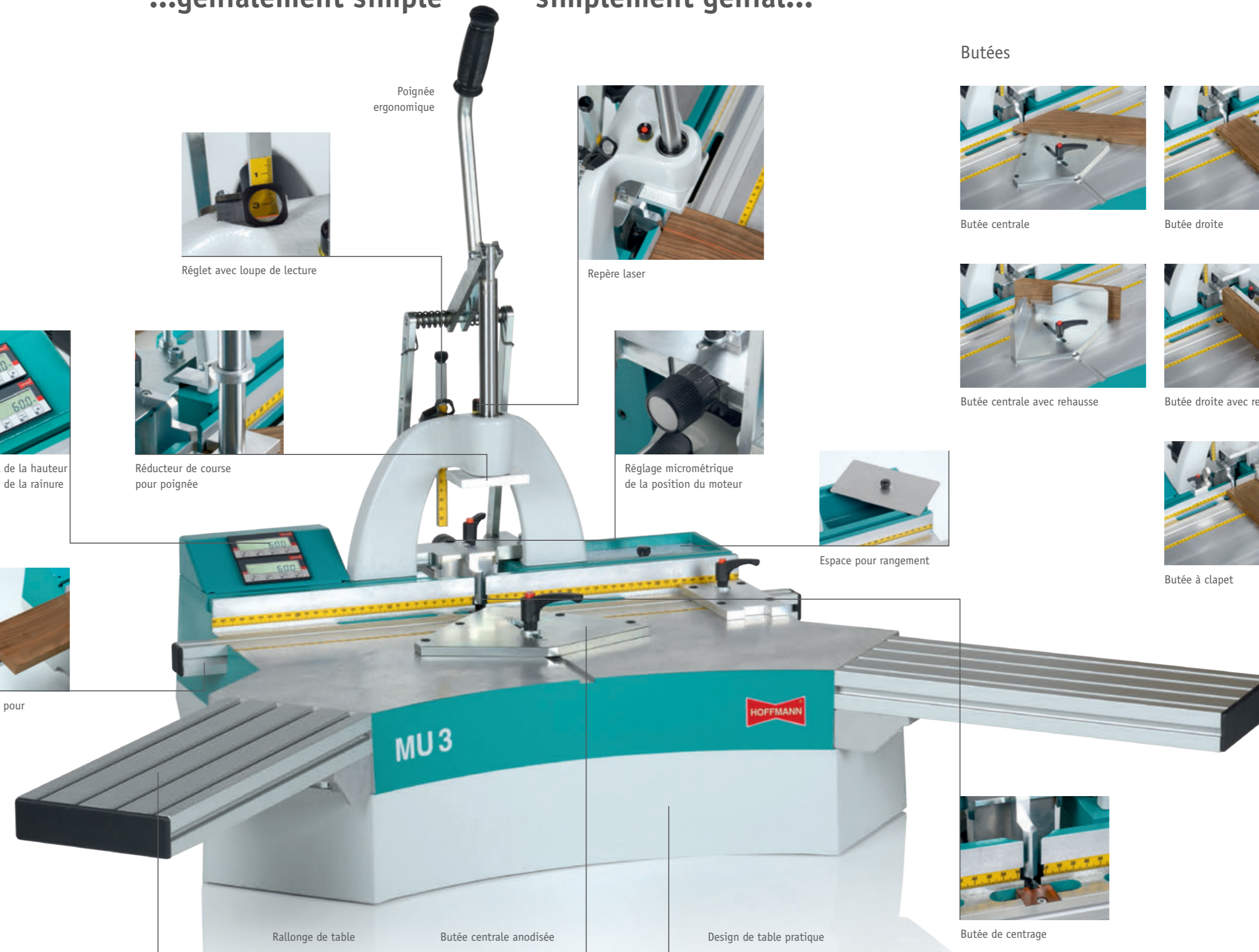
Rallonge de table
