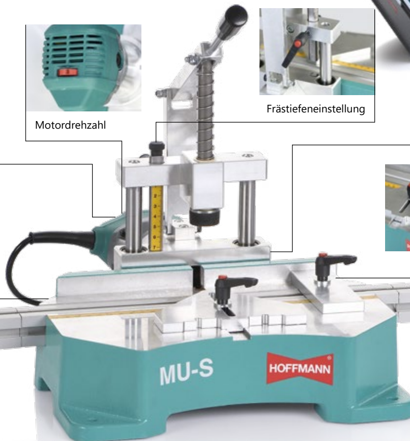
Fräshöheneinstellung
